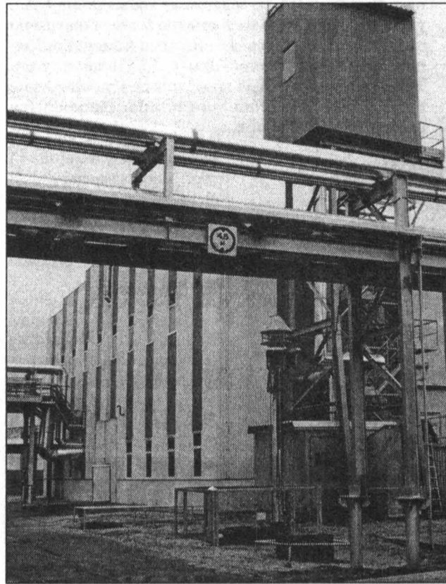
Здание ГТЭС на Конитлорском месторождении.
