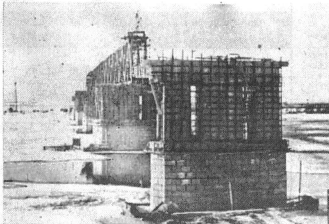
Строительство железнодорожного моста через Обь в районе Сургута.
